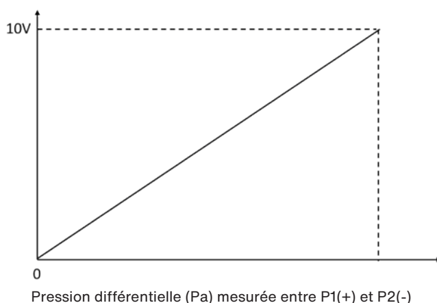
Transmetteur de pression TRPS/TRPR LOBBY
